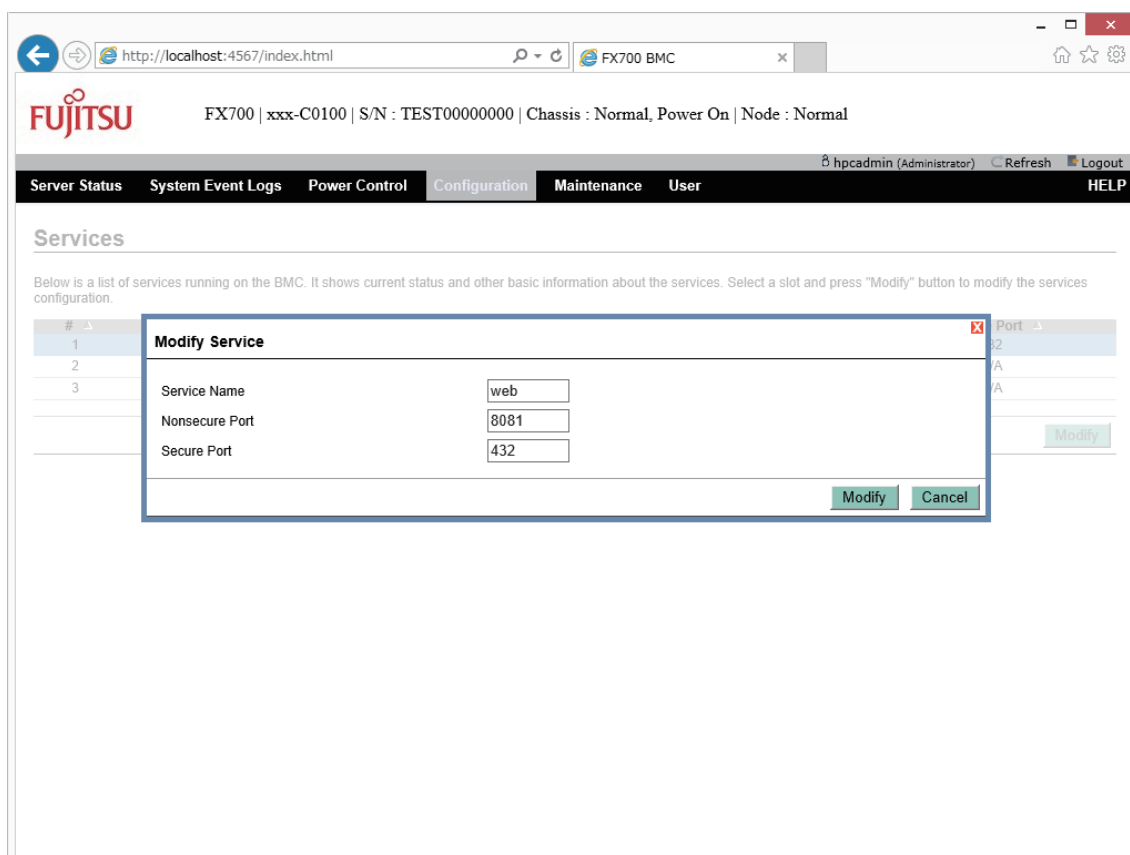
図 3.9 webサービス変更ダイアログボックス
