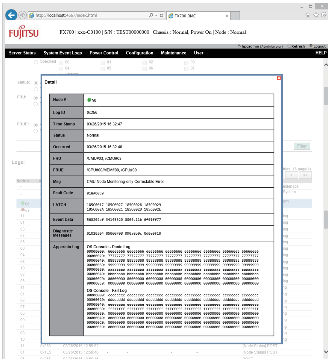
図 3.5 詳細ダイアログボックス
