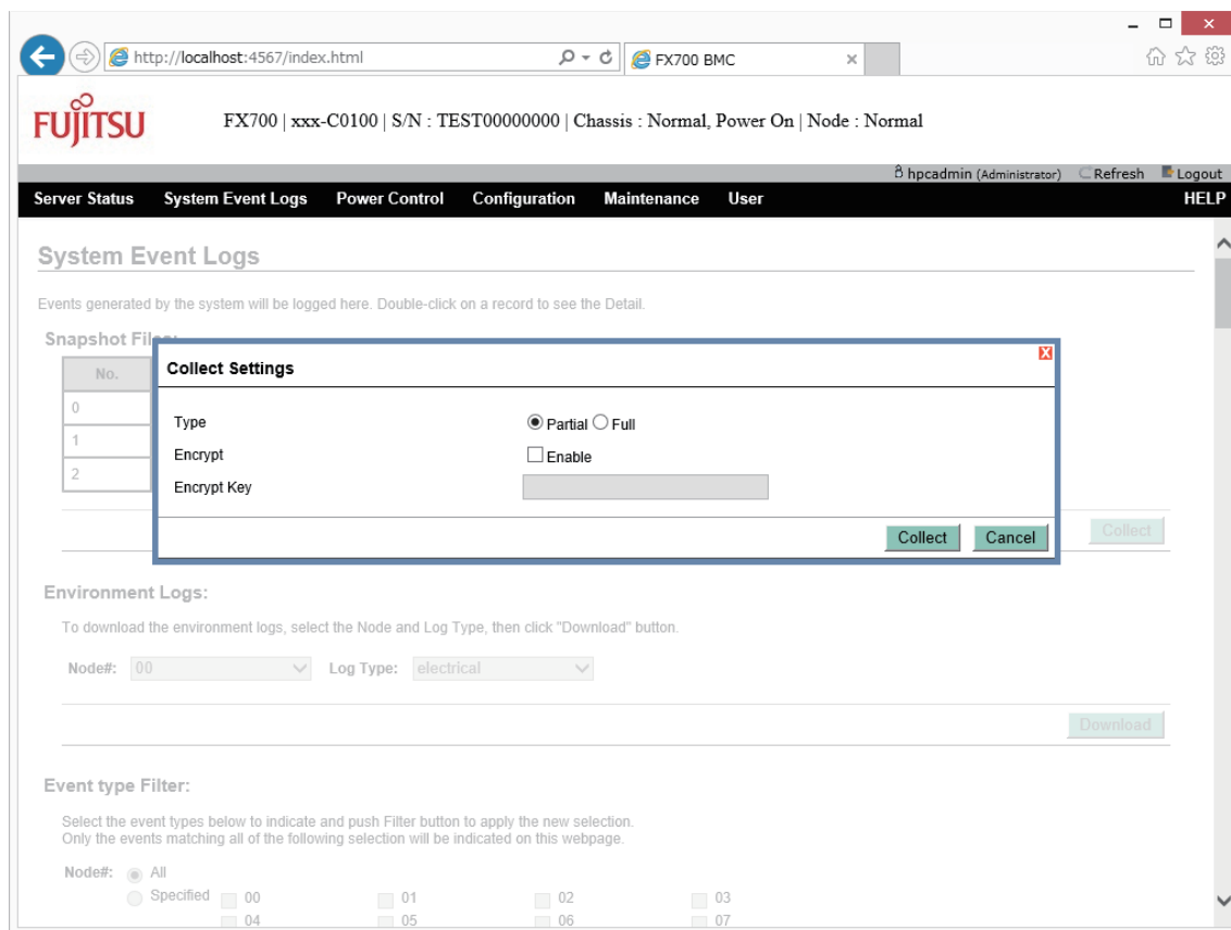
図 3.4 snapshot採取ダイアログ
