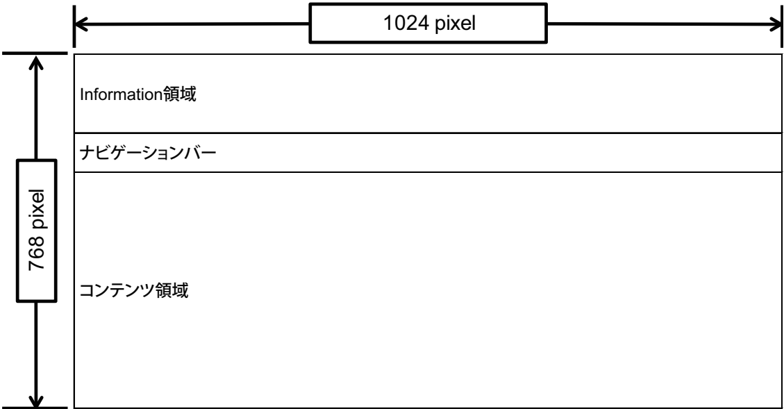
図 2.3 画面構成および画面サイズ
