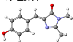
分子構造
