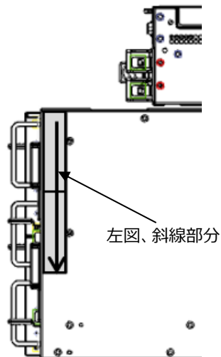
側面の拡大図(矢印は COA ラベル貼り付け方向)
