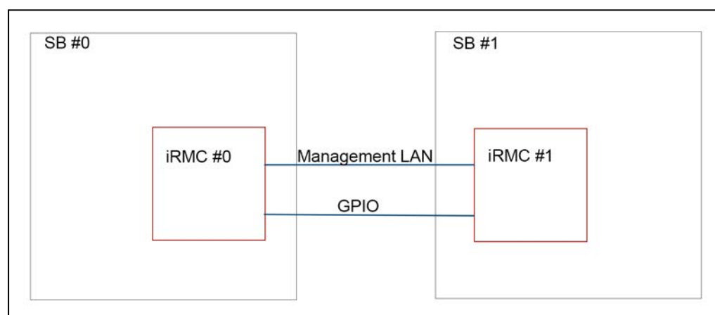
図 9: iRMC 間の通信
