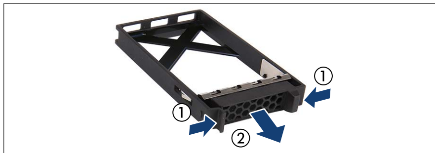
図 36: 2.5 インチ HDD/SSD ダミーモジュールの取り外し
