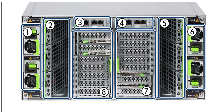
図 26: サーバの背面
