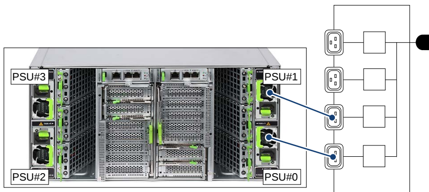
図 9: PSU 非冗長 (2+0) の配線図
