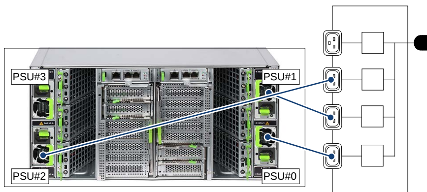
図 10: PSU 冗長 (2+1) の配線図
