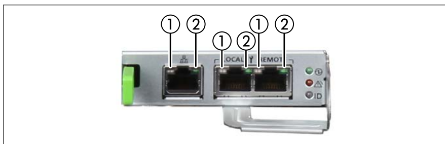
図 32: LAN 表示ランプ
