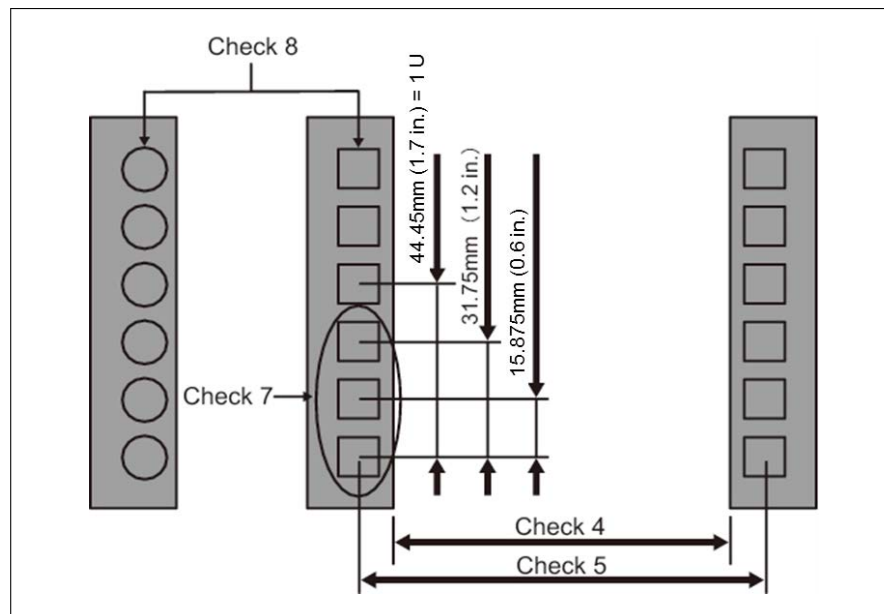
図 7: ラックポストの形式
