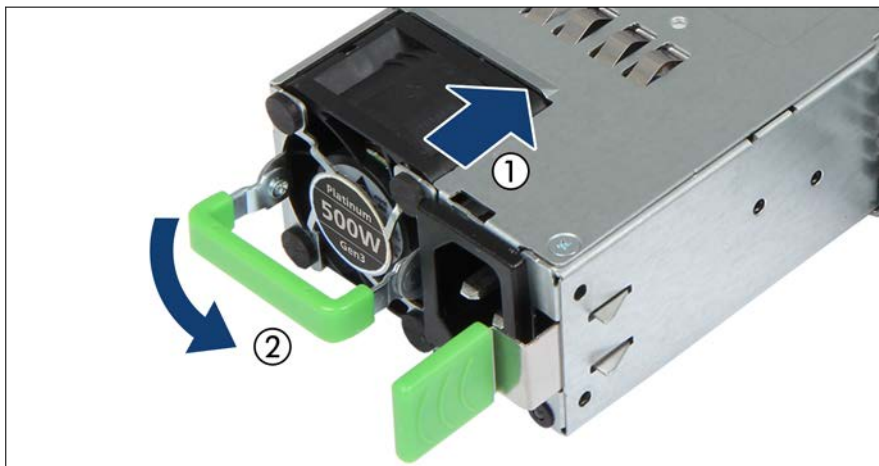
図 40: PSU の取り付け
