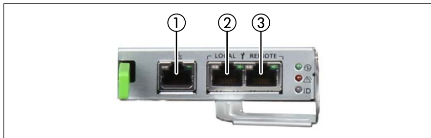
図 30: MLANU のコネクタ
