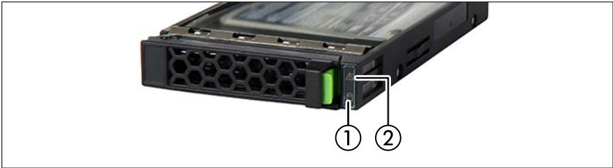
図 25: ホットプラグ PCIe SSD SFF モジュールの表示ランプ
