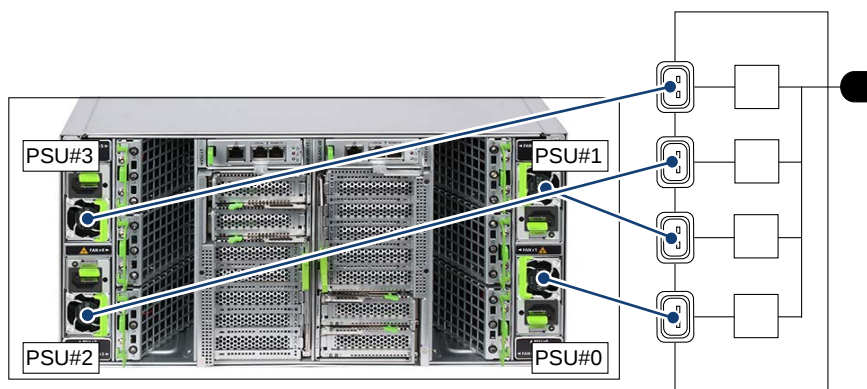
図 11: PSU 冗長 (2+2) の配線図
