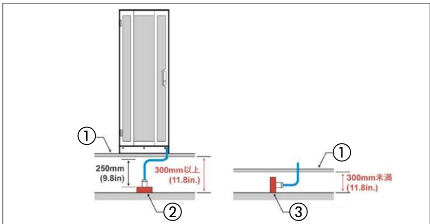
図 16: 上げ床の下での電源ケーブルの接続
