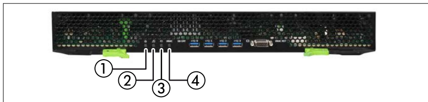
図 21: SB ユニットの表示ランプ
