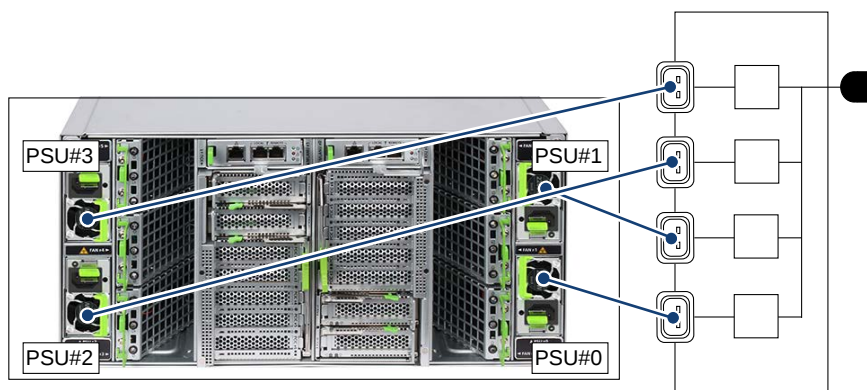
図 14: PSU 冗長 (3+1) の配線図
