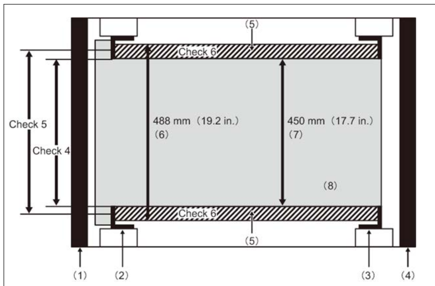
図 6: ラックの幅
