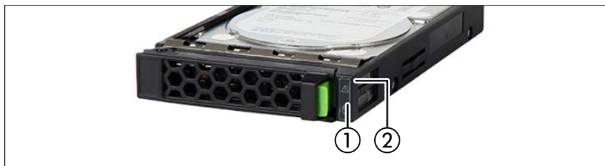
図 24: ホットプラグ SAS HDD/SSD モジュールの表示ランプ
