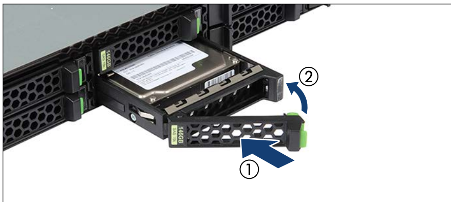
図 38: 2.5 インチ HDD/SSD モジュールの取り付け
