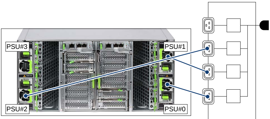
図 13: PSU 非冗長 (3+0) の配線図
