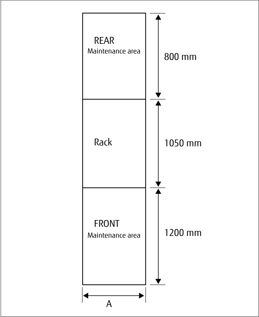
図 4: 設置エリア
