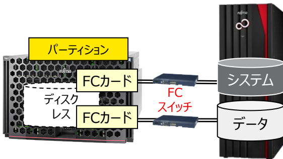
FCブート構成(*3)
