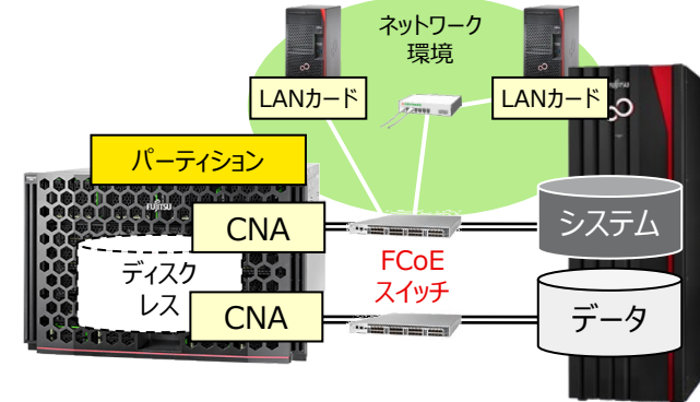
FCoEブート構成(*3)
