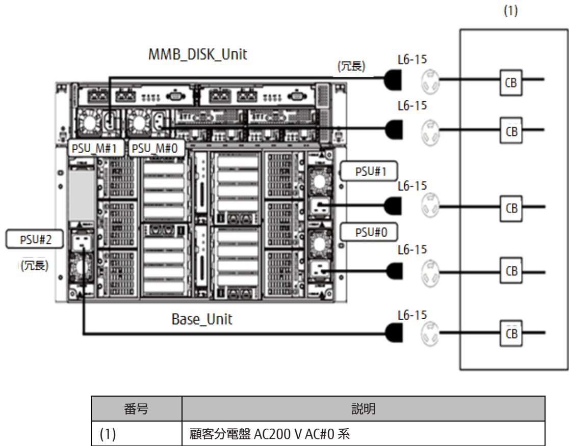
図 2.17 日本国内向け (標準) 200V 2+N : 電源非冗長(2+0)／電源冗長(2+1)
