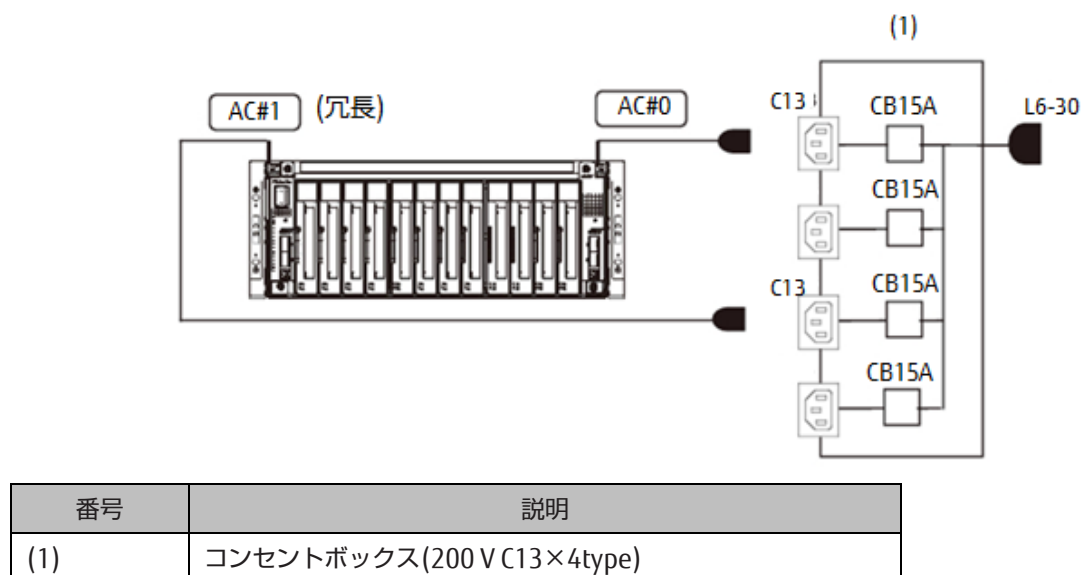
図 2.30 PCI ボックス日本国内向け／海外向け 200 V：電源非冗長／電源冗長(N+1/N+2)コンセントボックス接続
