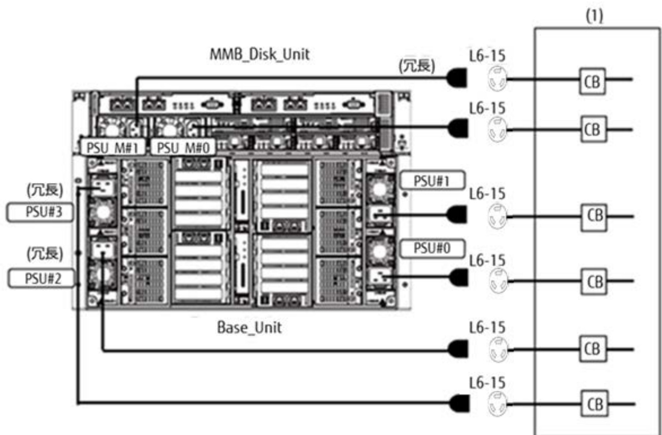
図 2.19 日本国内向け (標準) 200V 2+N : 電源冗長(2+2)
