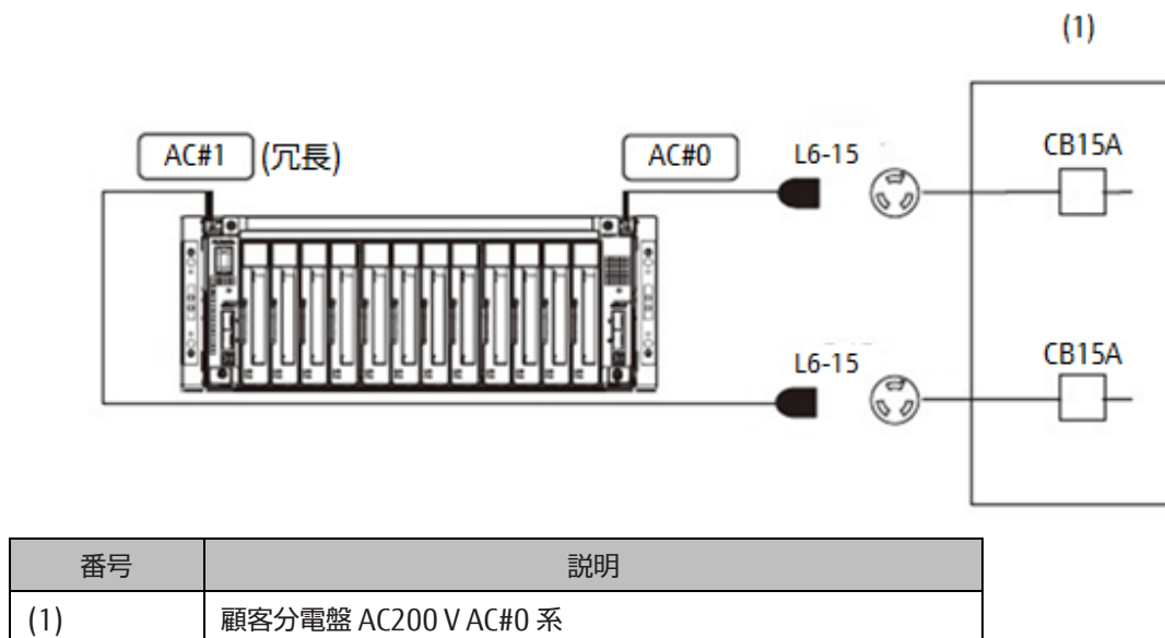
図 2.28 PCI ボックス日本国内向け 200 V : 電源非冗長／電源冗長(N+1/N+2)
