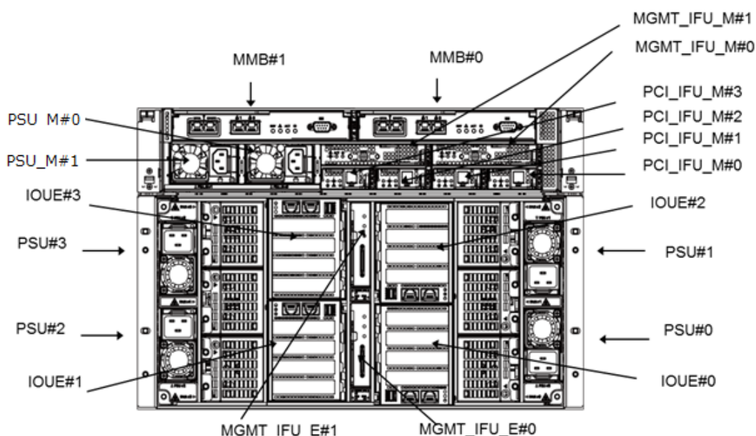
図 2.8 外部インターフェース接続部(PRIMEQUEST 3400E2/3400L2/3800E2/3800L2/3400E/3400L/3800E/3800L (背面))
