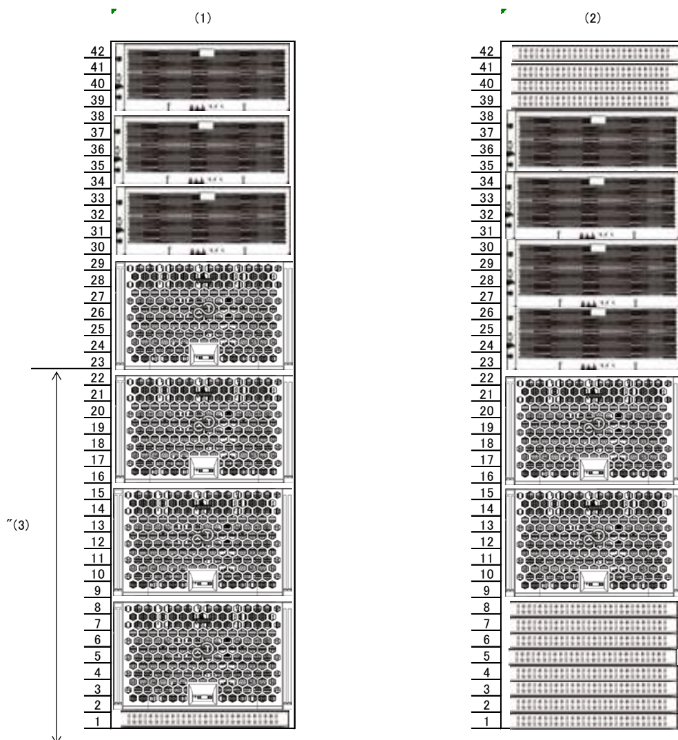
図 A.1 ラック搭載例
