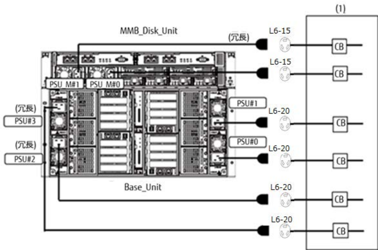
図 2.18 日本国内向け (高出力) 200V 2+N : 電源冗長(2+2)
