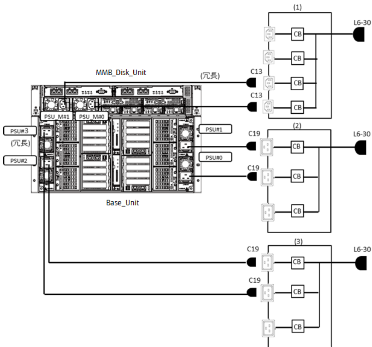
図 2.23 日本国内向け／海外向け (高出力／標準) 200V 2+N : 電源冗長(2+2) コンセントボックス接続
