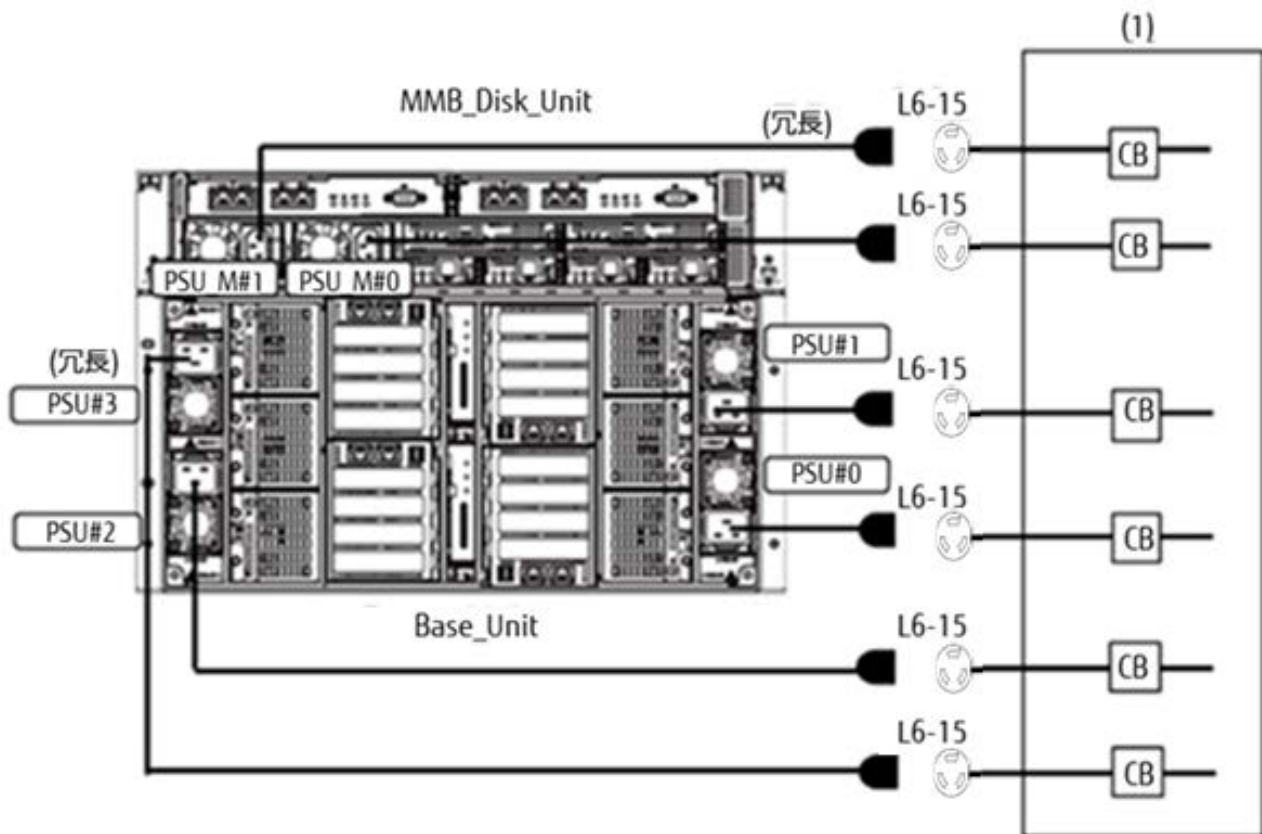
図 2.25 日本国内向け 200V 3+N: 電源非冗長(3+0)／電源冗長(3+1)
