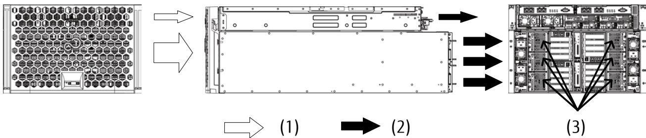
図 1.10 冷却風および排気の流れ(本体装置)
