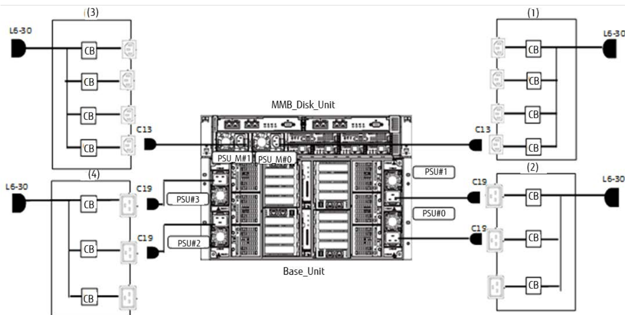
図 2.24 日本国内向け／海外向け (高出力 PSU／標準 PSU) 200V 2+N : 電源二系統 コンセントボックス接続
