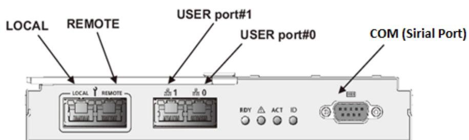
図 2.9 外部インターフェース詳細(MMB)
