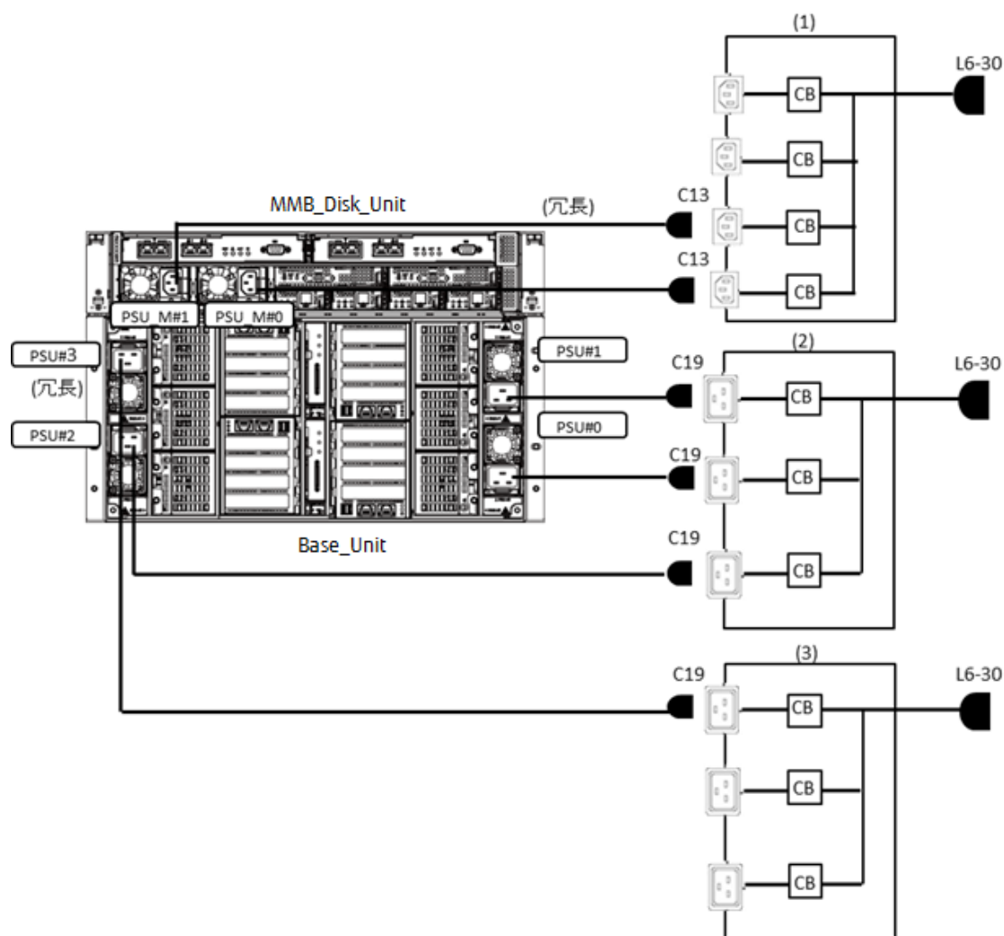
図 2.26 日本国内向け／海外向け 200V 3+N：電源非冗長(3+0)／電源冗長(3+1)コンセントボックス接続
