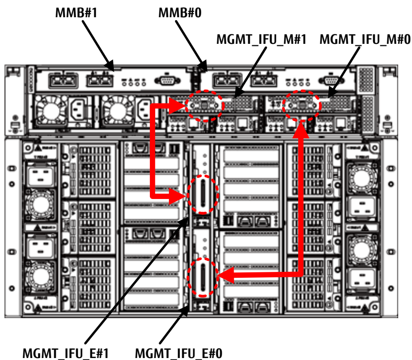
図 2.2 MGMT_IFU_E と MGMT_IFU_M の接続
