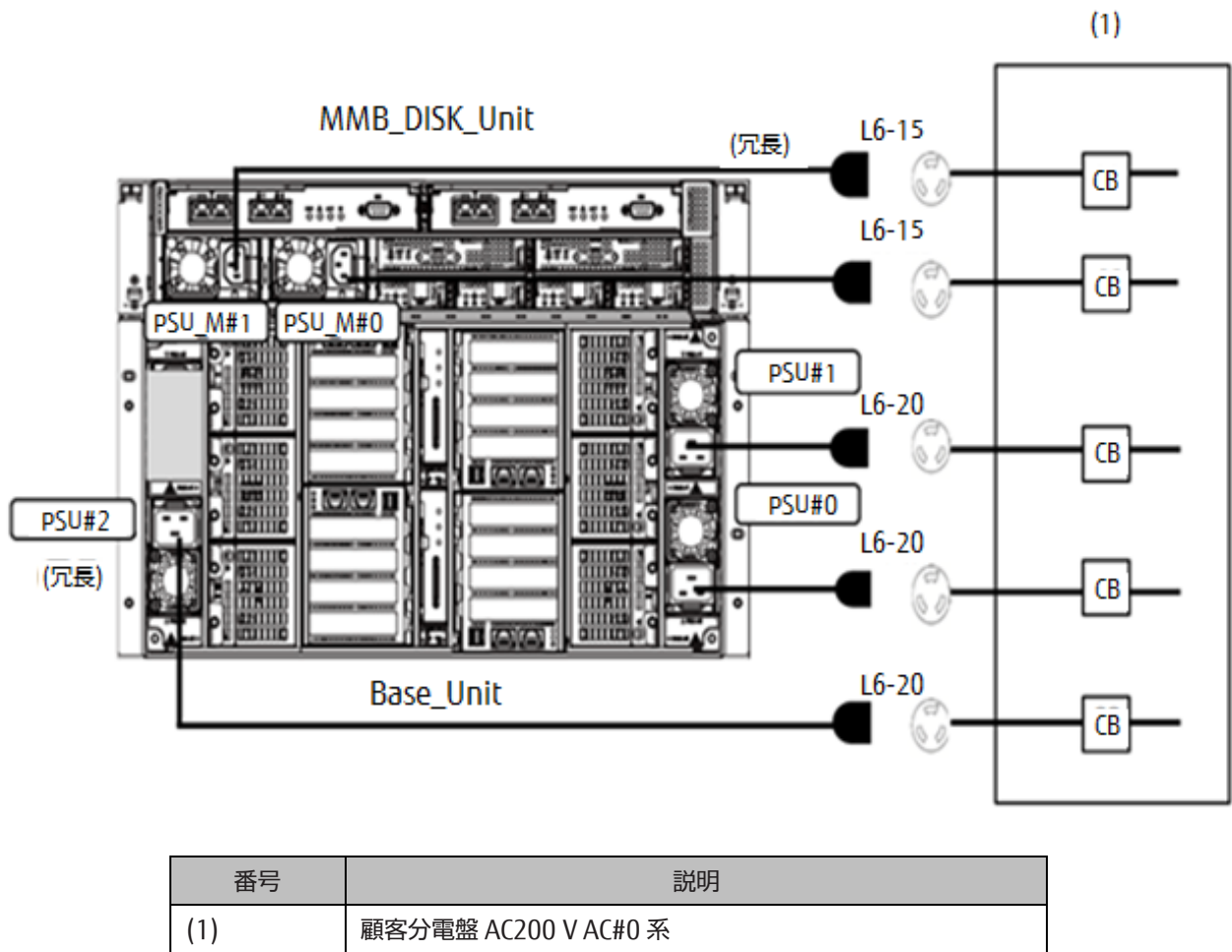
図 2.16 日本国内向け (高出力) 200V 2+N : 電源冗長(2+1)
