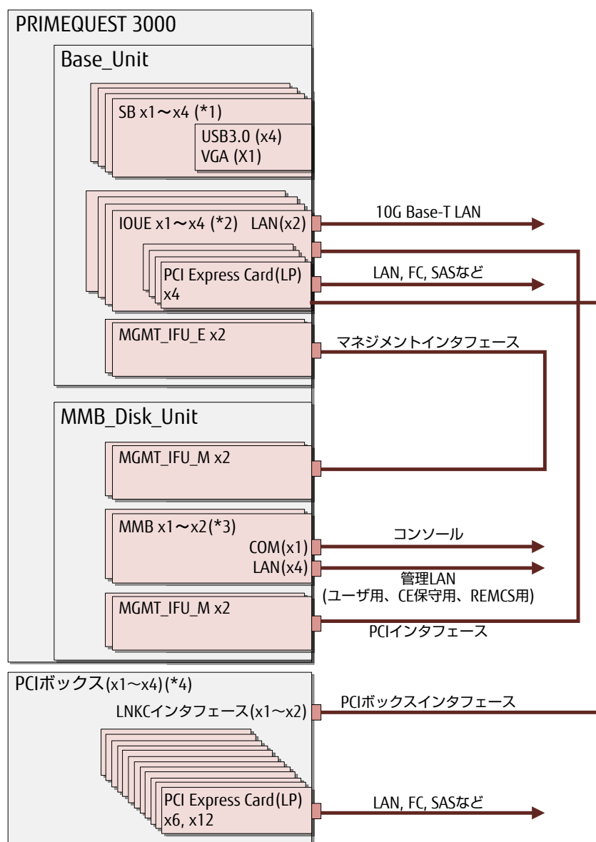
図 2.1 装置接続の概要
