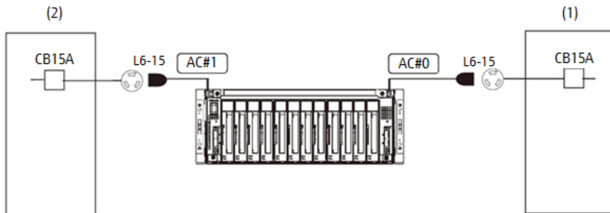
図 2.29 PCI ボックス日本国内向け 200 V : 電源二系統
