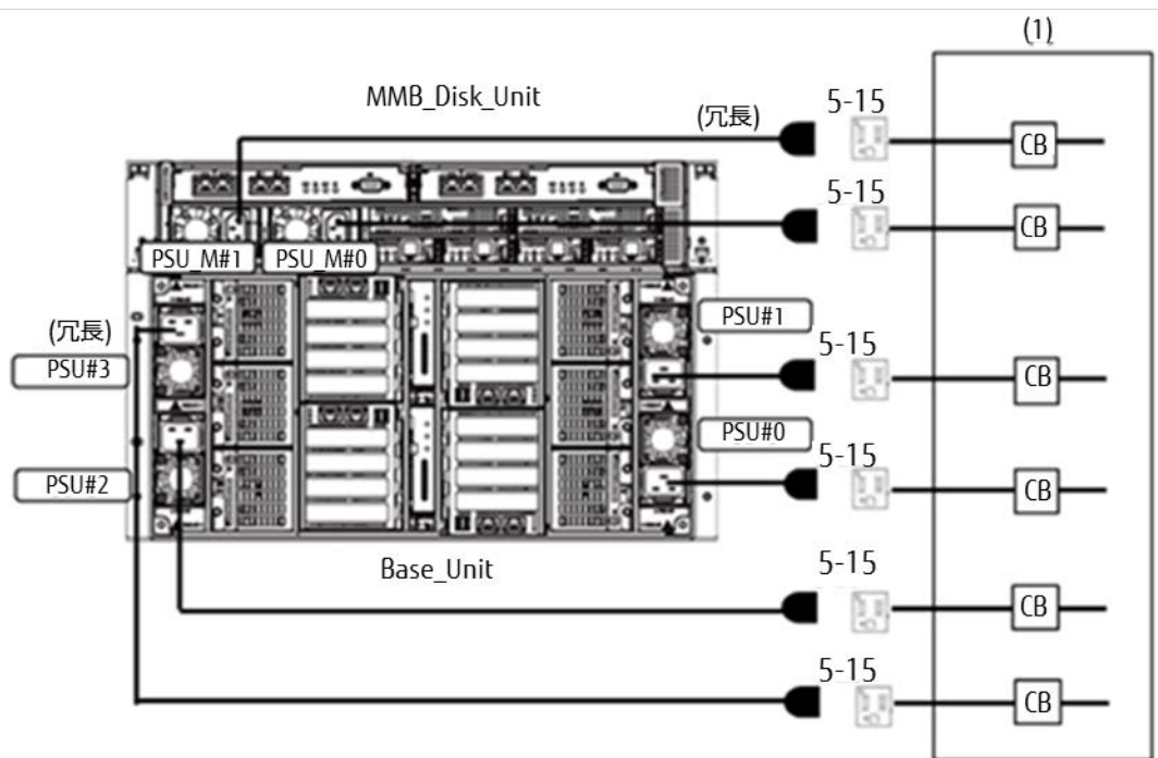
図 2.15 日本国内向け／海外向け 100 V：電源非冗長／電源冗長(3+1)
