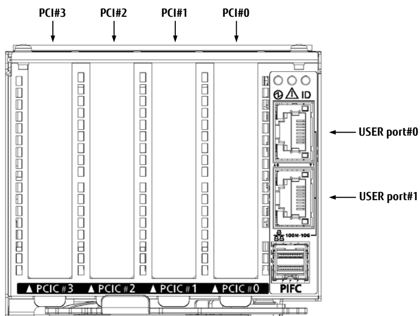
図 2.10 外部インターフェース詳細(IOUE)
