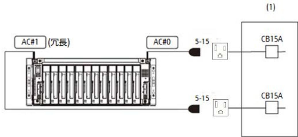
図 2.27 PCI ボックス日本国内向け／海外向け 100 V：電源非冗長／電源冗長(N+1)
