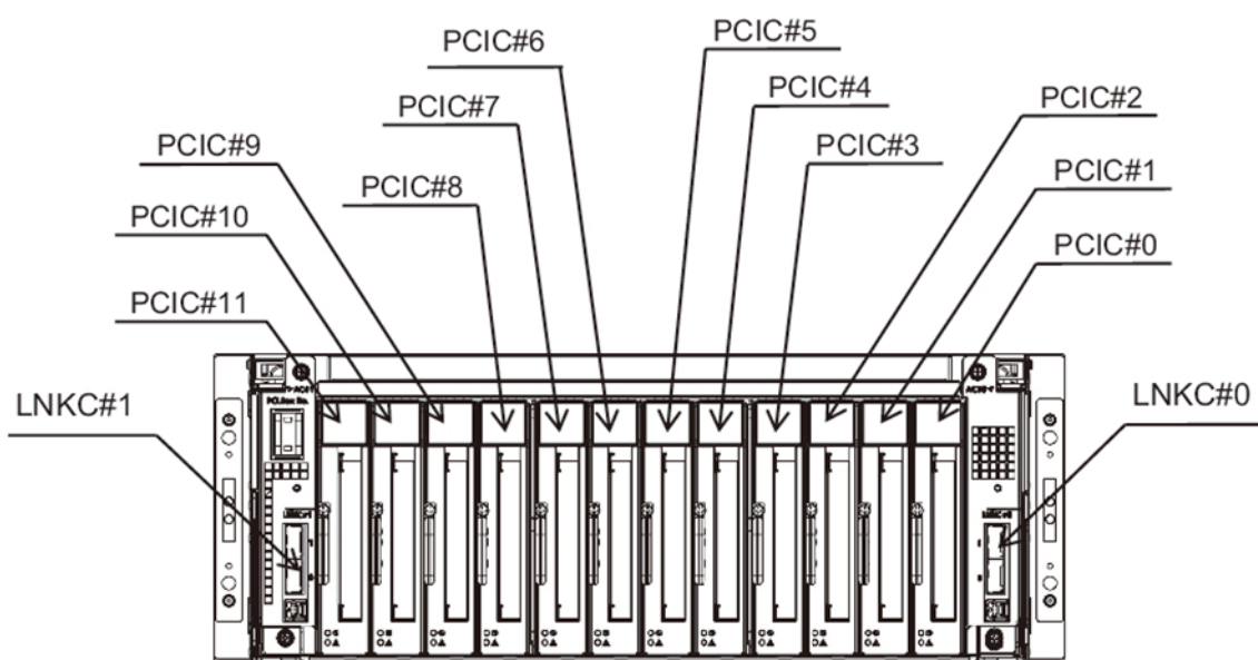
図 2.14 外部インターフェース詳細(PCI ボックス)
