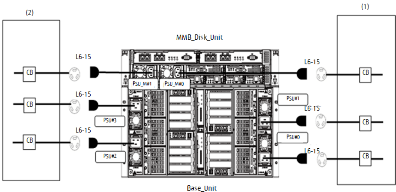
図 2.21 日本国内向け (標準)200V 2+N : 電源二系統
