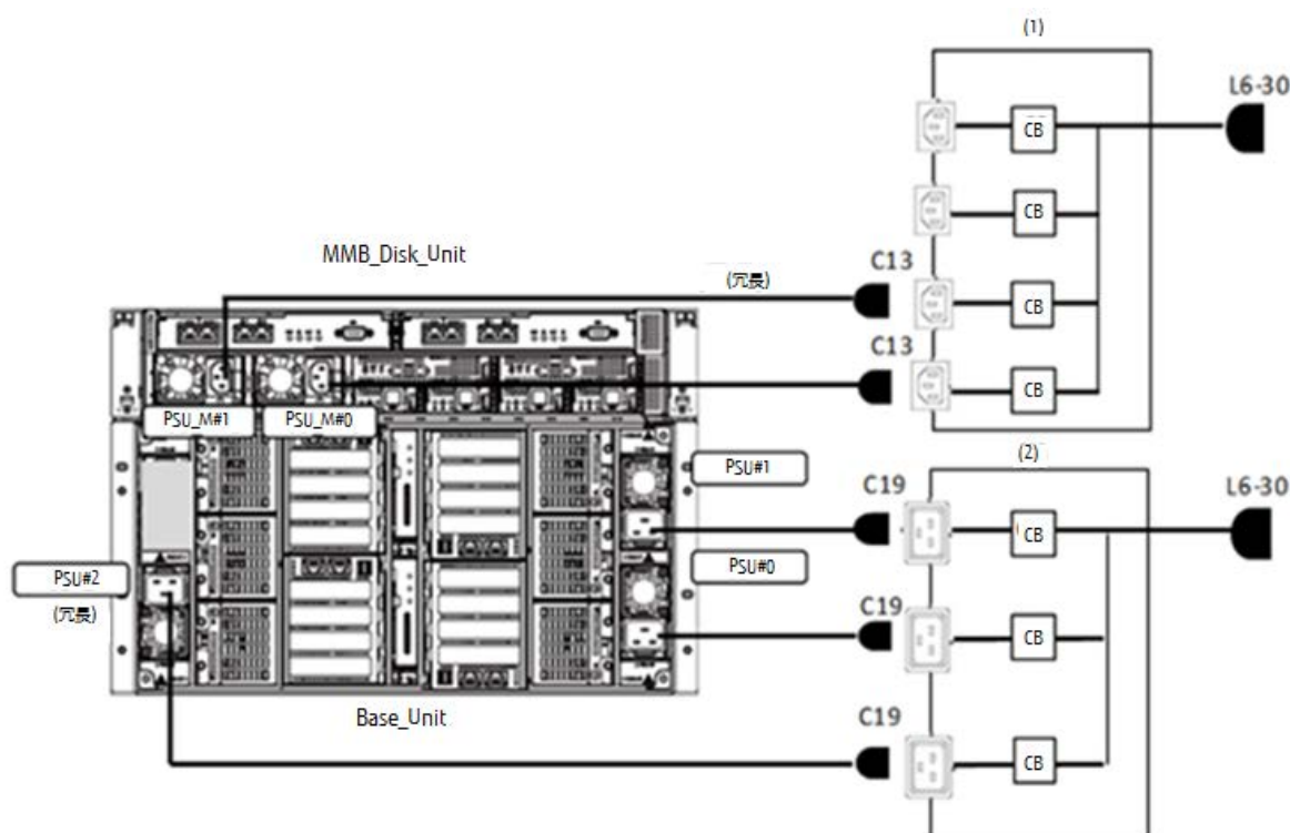
図 2.22 日本国内向け／海外向け (高出力／標準) 200V 2+N : 電源非冗長(2+0)／電源冗長(2+1)コンセントボックス接続
