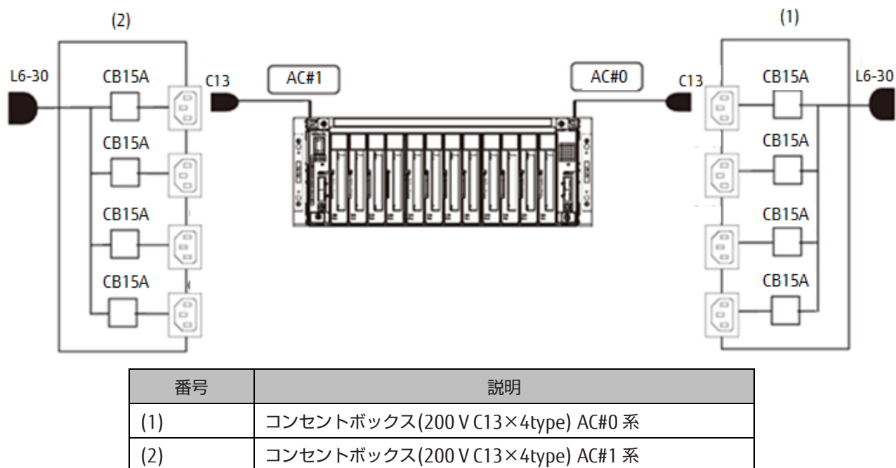
図 2.31 PCI ボックス日本国内向け／海外向け 200 V：電源二系統コンセントボックス接続
