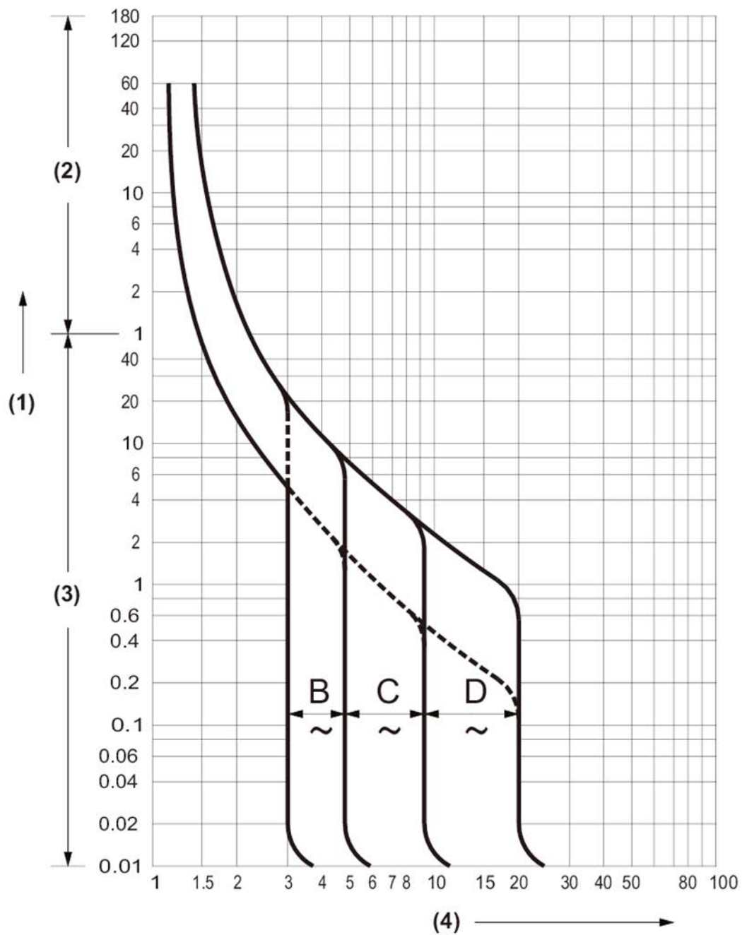
図 2.34 分電盤のブレーカ特性
