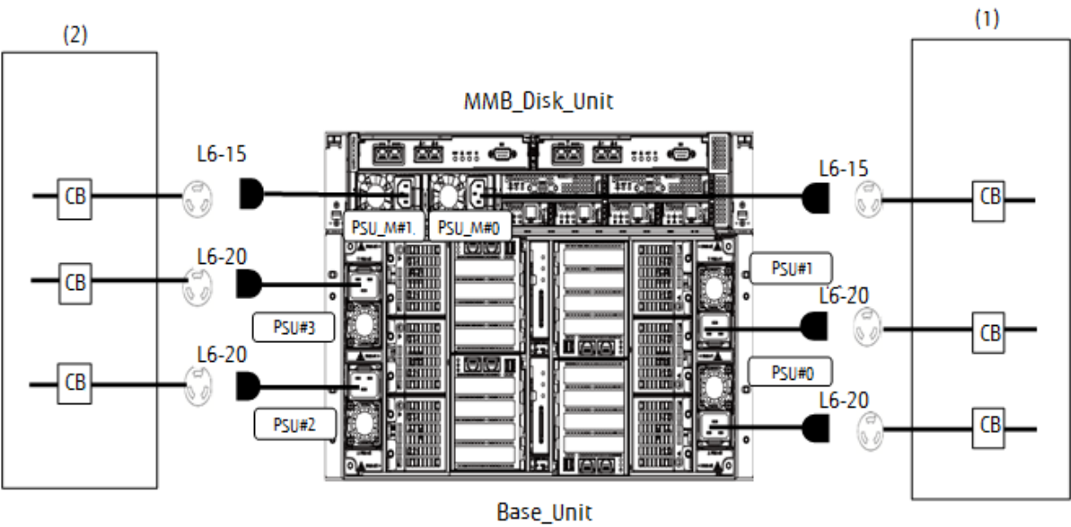
図 2.20 日本国内向け (高出力) 200V 2+N : 電源二系統
