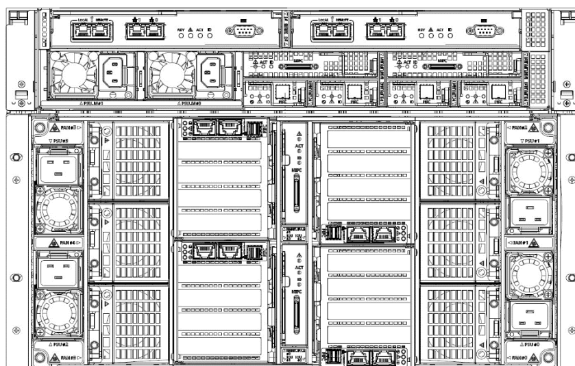
図 1.2 本体装置背面
