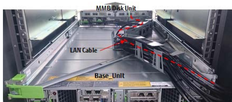
図 2.4 装置背面(MMB_Disk_Unit を前面へ引き出した状態)
