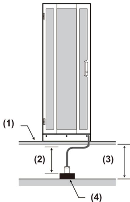
図 2.33 床下の高さが 300 mm (11.8 in.)以上の場合
