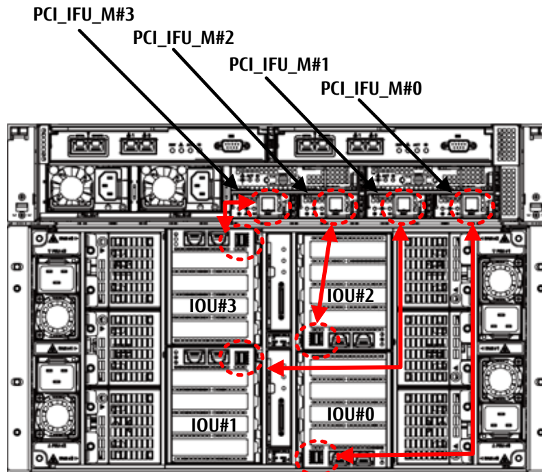
図 2.3 IOUE と PCI_IFU_M の接続
