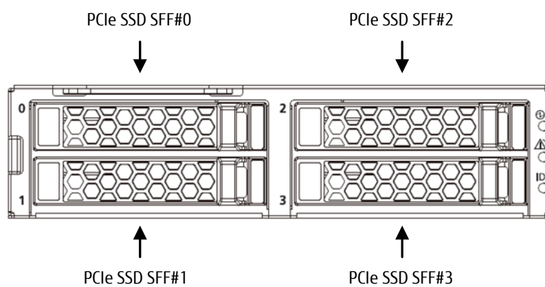
図 2.12 外部インターフェース詳細(DU_PCIEA)
