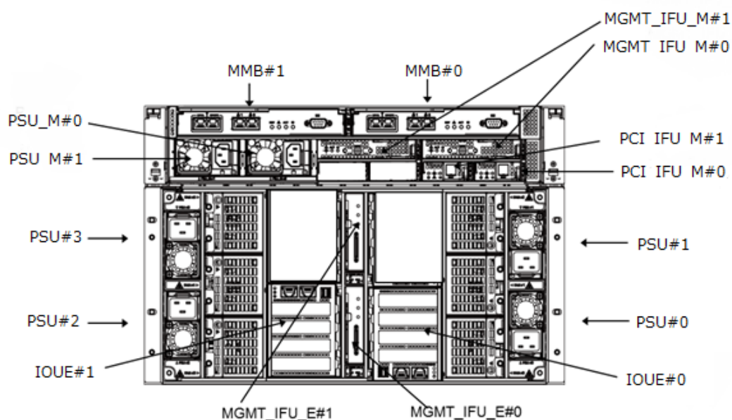
図 2.6 外部インターフェース接続図(PRIMEQUEST 3400S2 Lite/3400S2/3400S Lite/3400S (背面))
