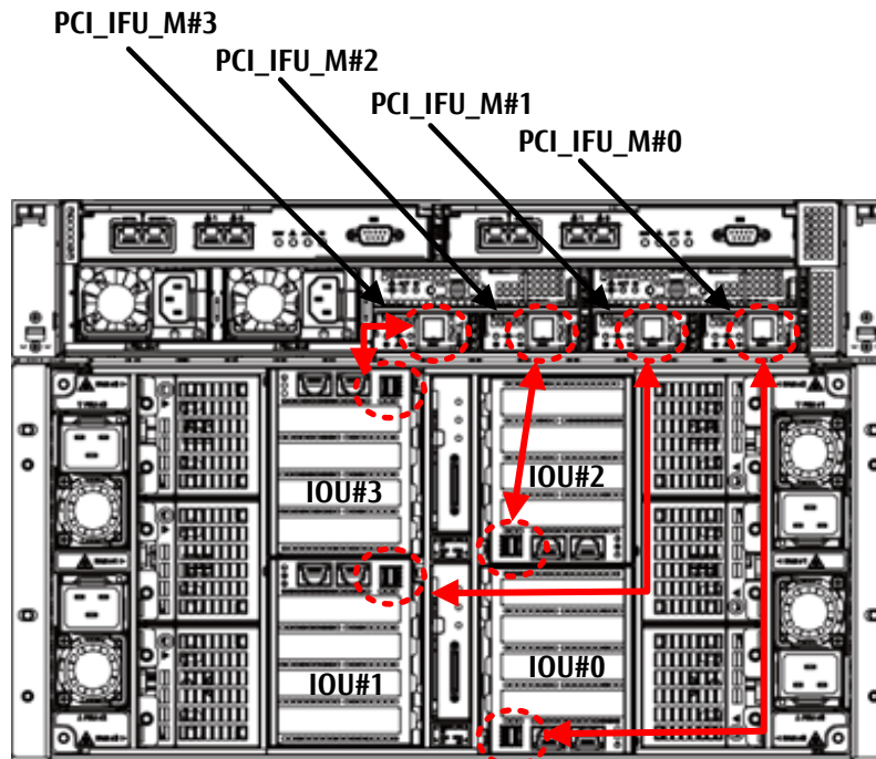
図 2.3 IOUE と PCI_IFU_M の接続
