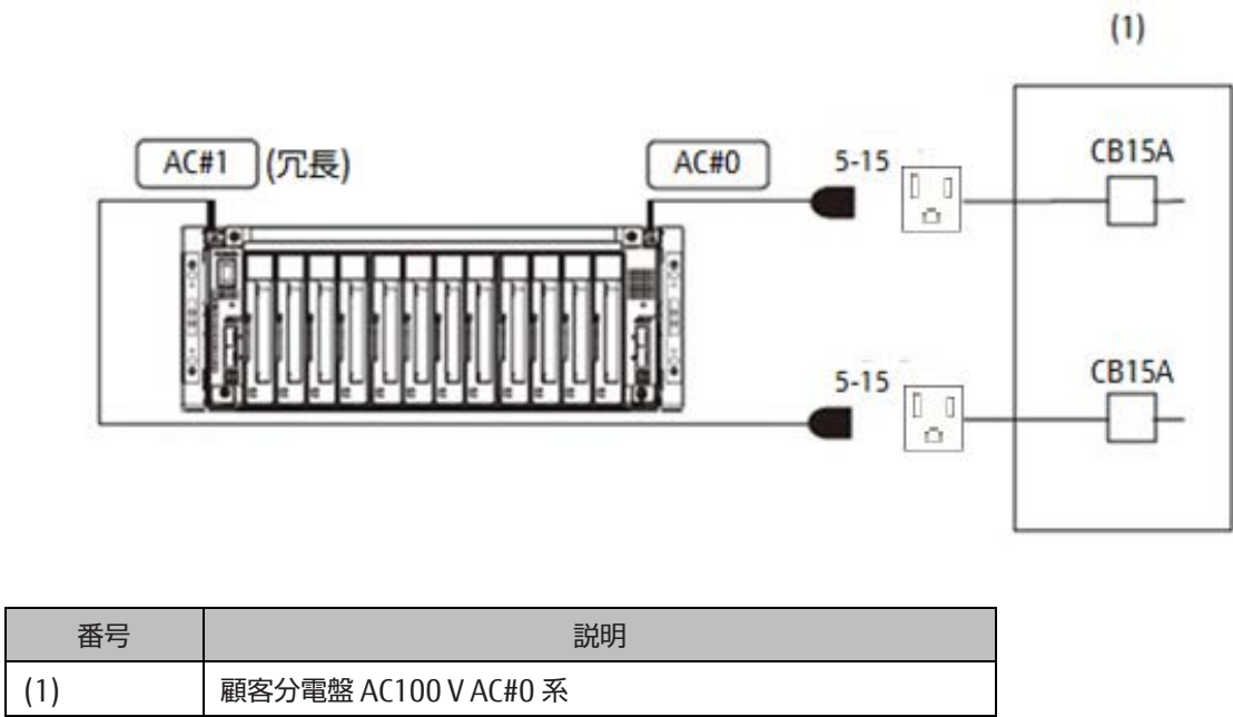
図 2.27 PCI ボックス日本国内向け／海外向け 100 V：電源非冗長／電源冗長(N+1)
