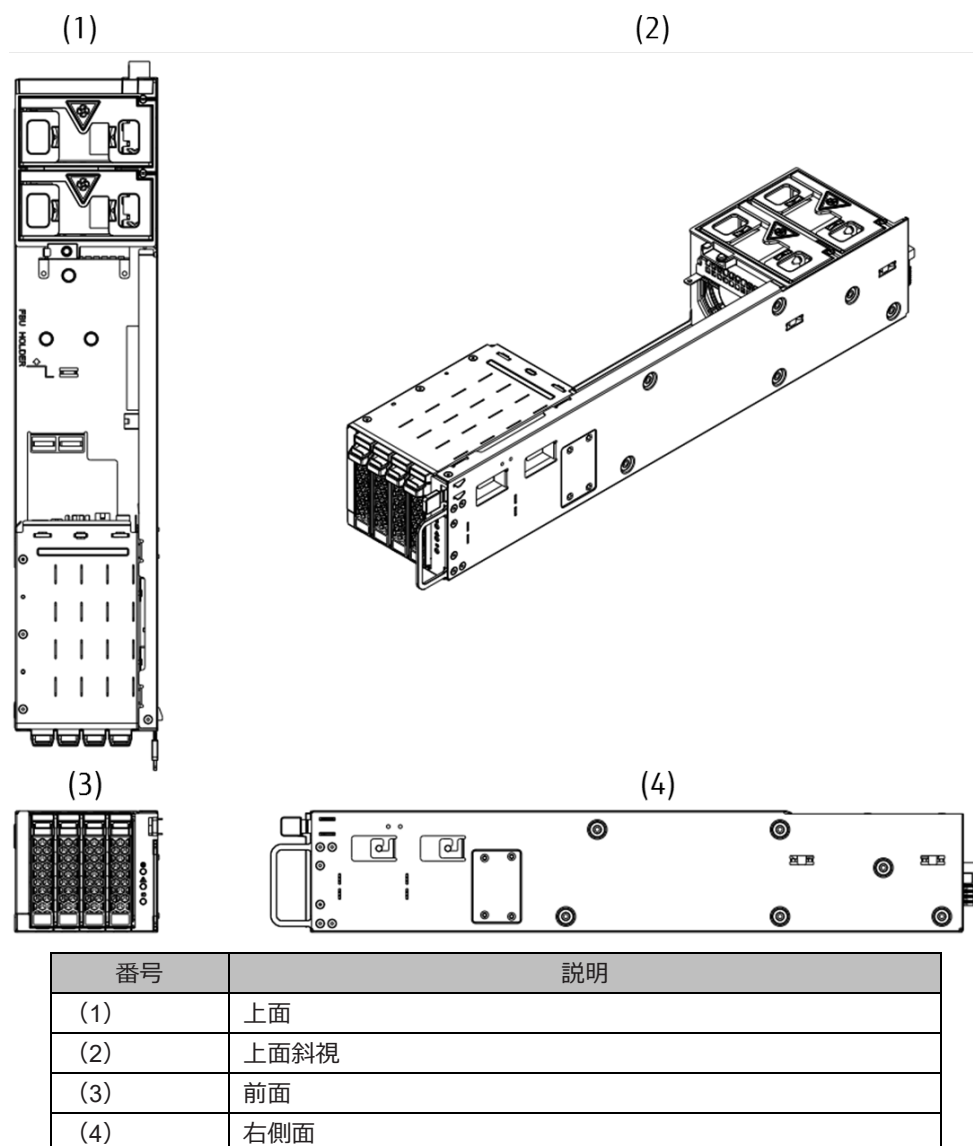
図 2.15 DU_M の外観図
