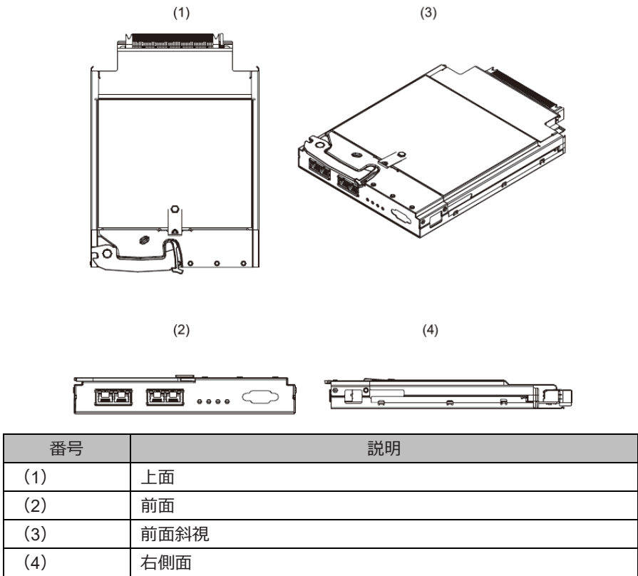
図 2.8 MMB 外観図
