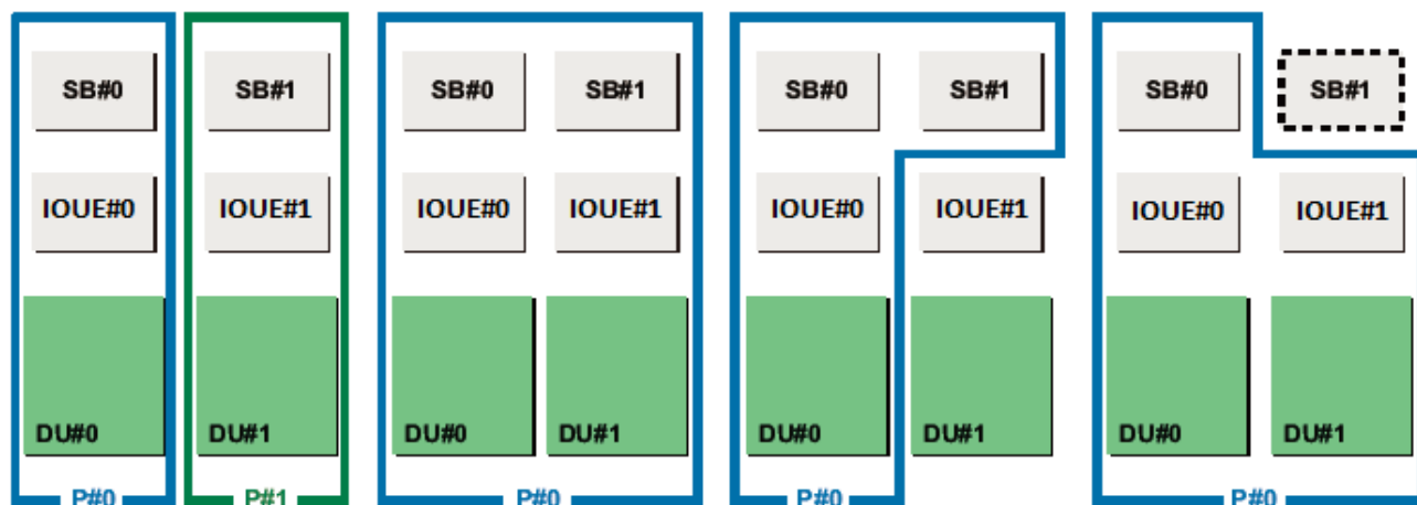
図 5.2 パーティショニング機能の概念図（PRIMEQUEST 3400E2/3400L2/3400E/3400L）
