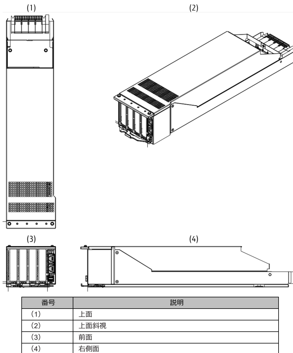
図 2.9 IOUE 外観図
