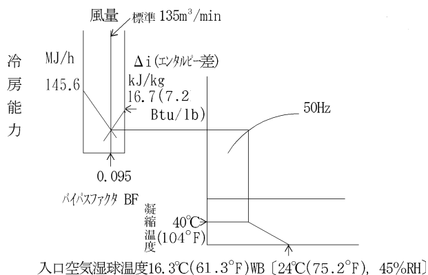
図 4.7 パッケージ空調設備の特性例
