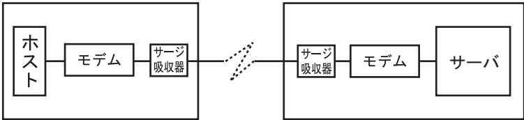
図 7.3 外付けモデム使用時の避雷対策
