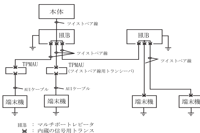
図 6.7 100Base-T の代表的な接続形態
