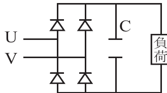
図 6.5 整流負荷回路
