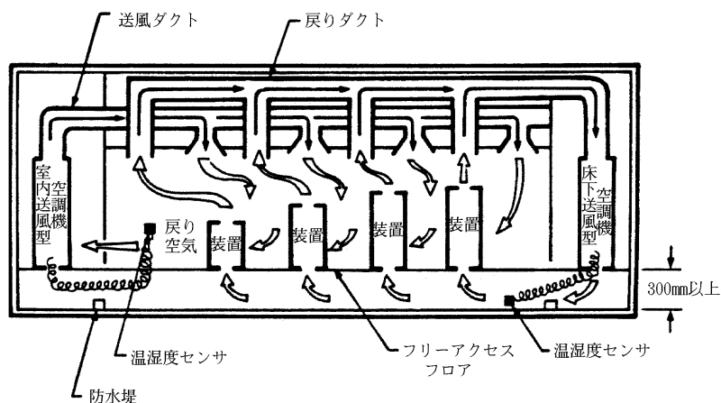
図 4.4 室内空調と床下送風方式の併用
