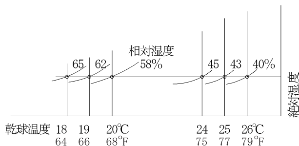
図 4.5 室内温度を変えるときの空気線図
