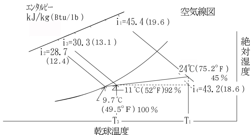
図 4.8 空気線図上の空気状態（パッケージ空調設備の例）
