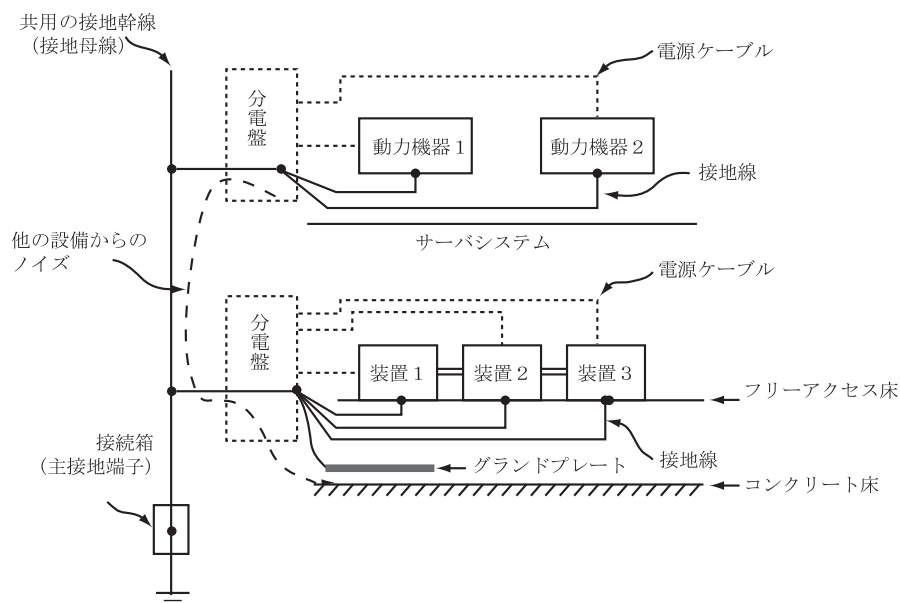
図 6.8 グラウンドプレート工法
