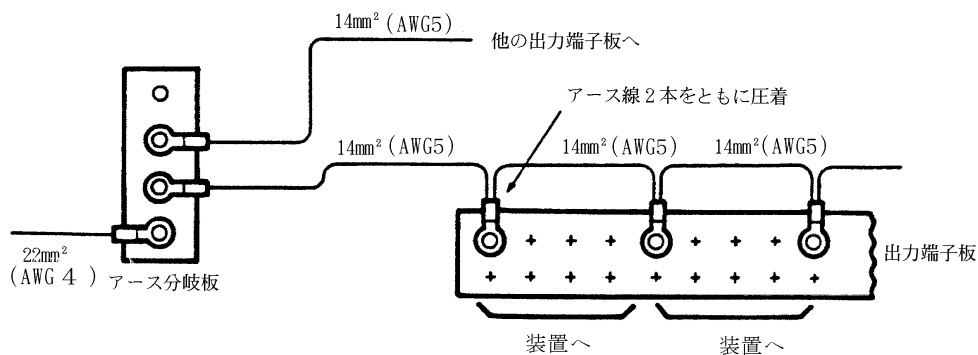
図 6.13 分電盤内のアース接続
