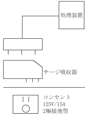
図 7.1 コンセント差し込み型のサージ吸収器
