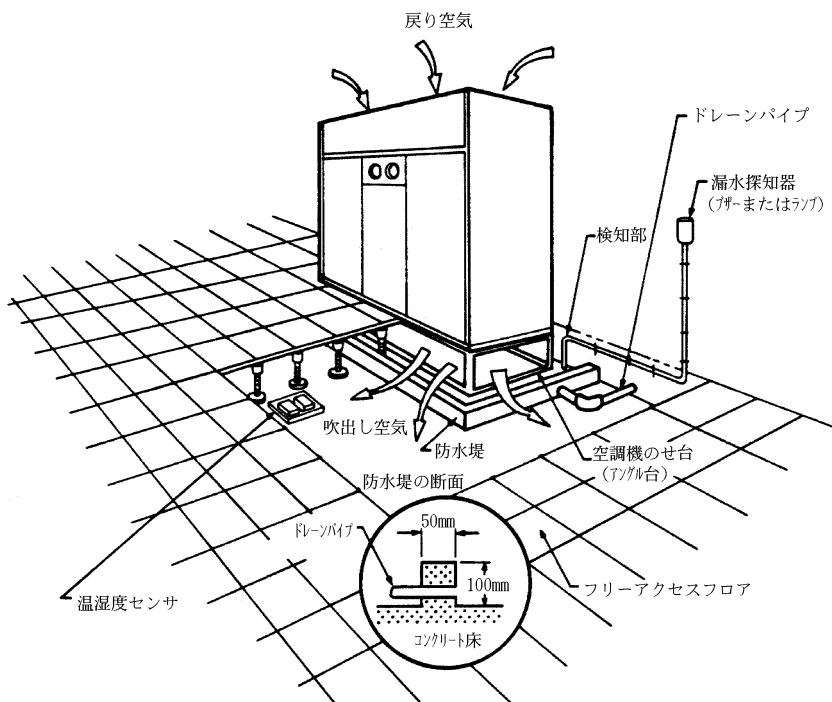
図 4.10 防水堤
