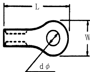
図 6.11 丸型圧着端子の寸法
