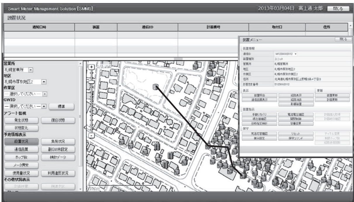
図-4 検針ネットワークの可視化
