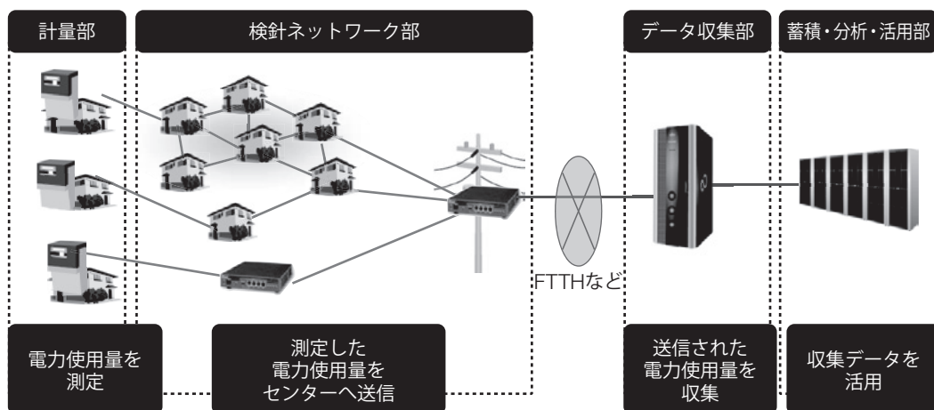
図-1 スマートグリッド構成概要
