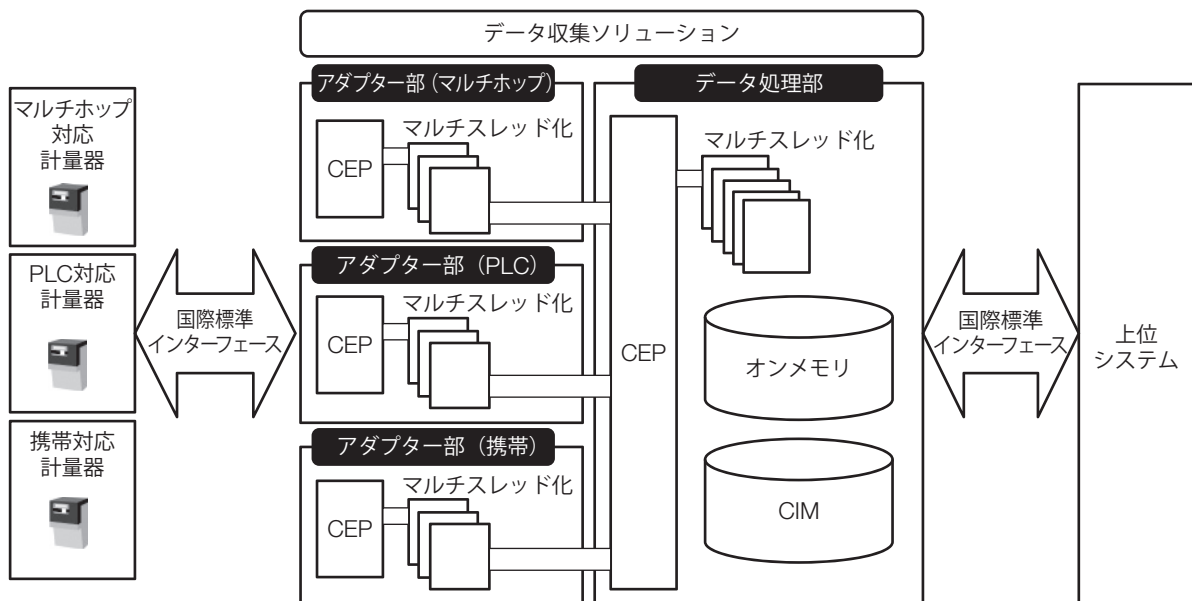
図-3 データ収集ソリューションの構成と機器・システム間インターフェース
