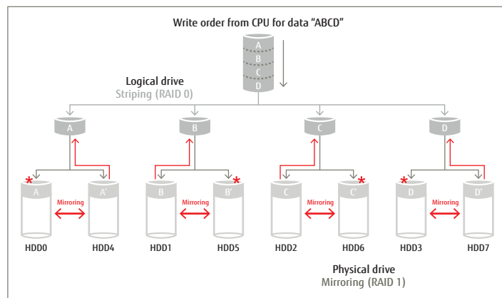
RAID 1+0
