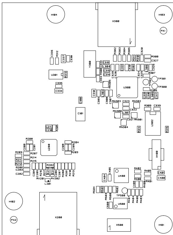
Fujitsu Jade Evaluation Board Extension Video Out PA5 Datum: 07.12.2007 Bestückungsplan Top
