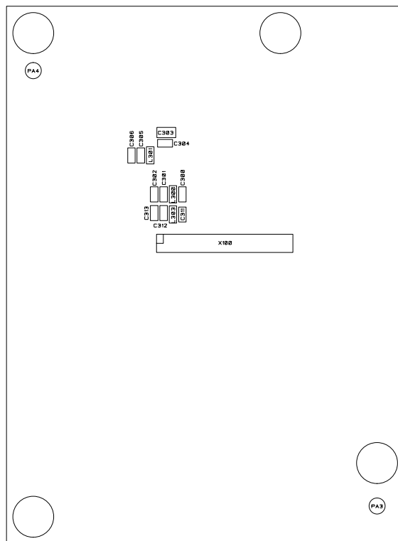
Fujitsu Jade Evaluation Board Extension Video Out PA5 Datum: 07.12.2007 Bestückungsplan Bottom
