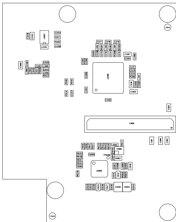
Fujitsu JADE Evaluation Board Extension Video Input PA5 Datum: 27.08.2007 Bestückungsplan Bottom
