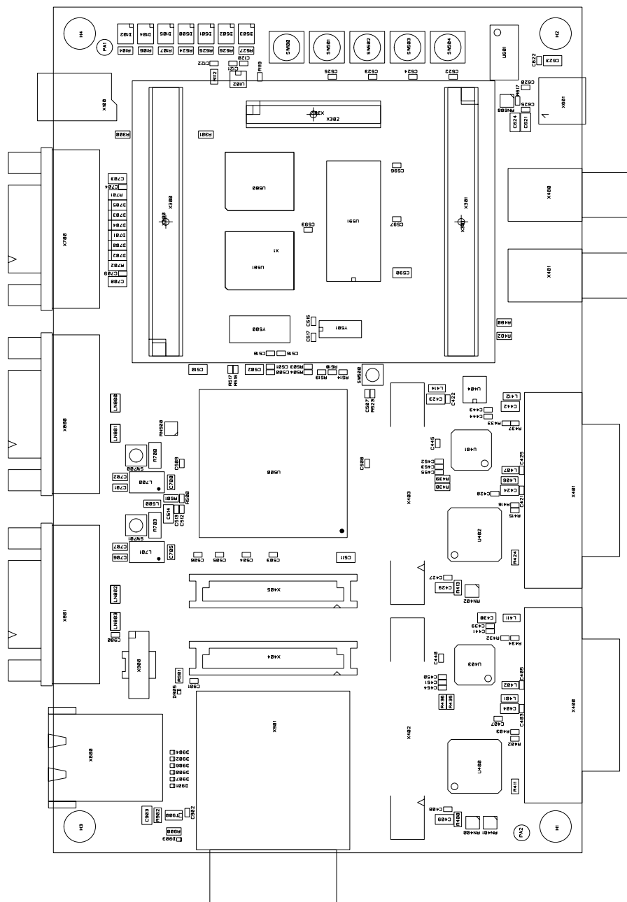
467/GDC-Board PA3 Bestückungsplan Top Datum: 04.10.2007
