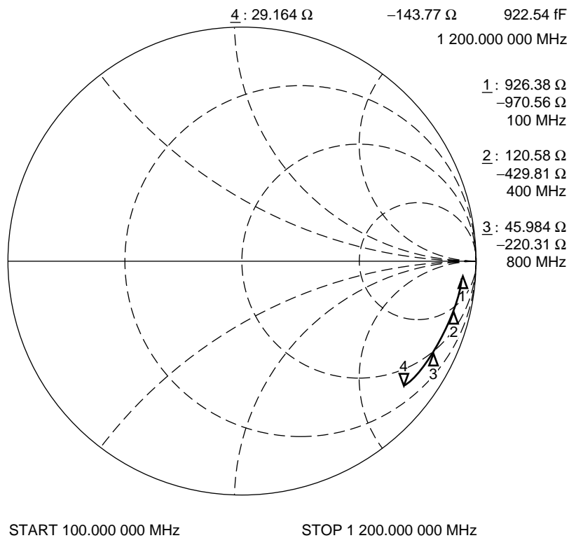
fin IF input impedance
