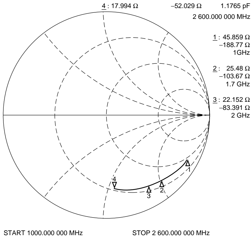
fin RF input impedance
