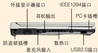
左视图
